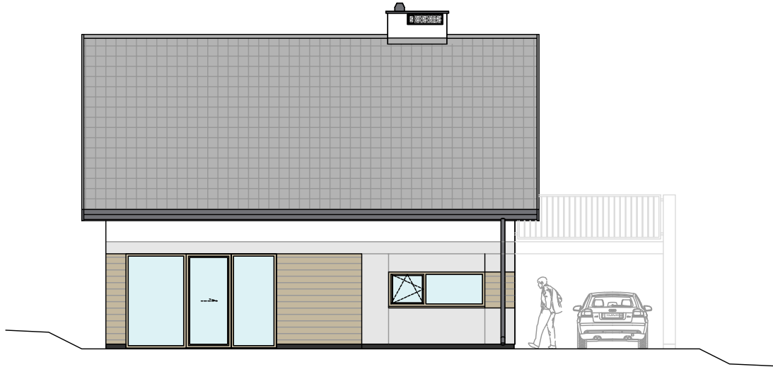
ELEWACJA POŁUDNIOWA
