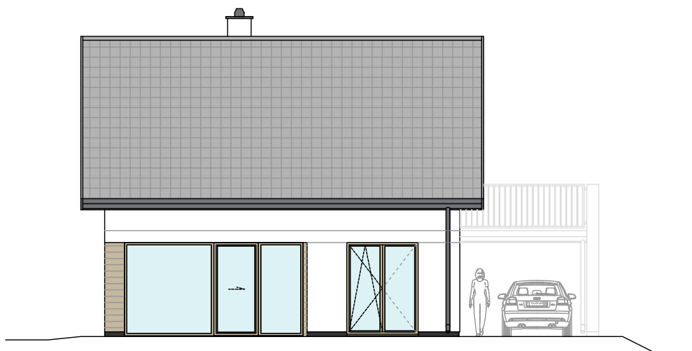
ELEWACJA POŁUDNIOWA
