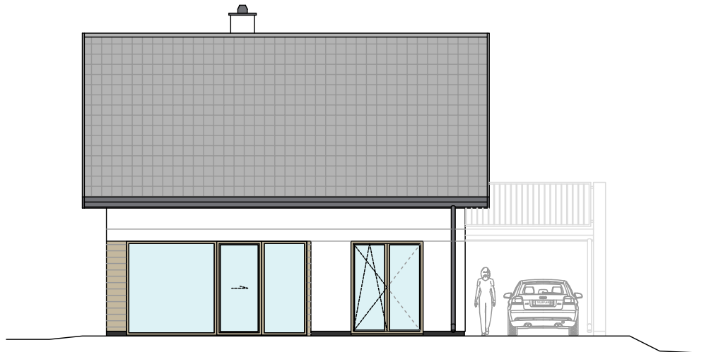
ELEWACJA POŁUDNIOWA
