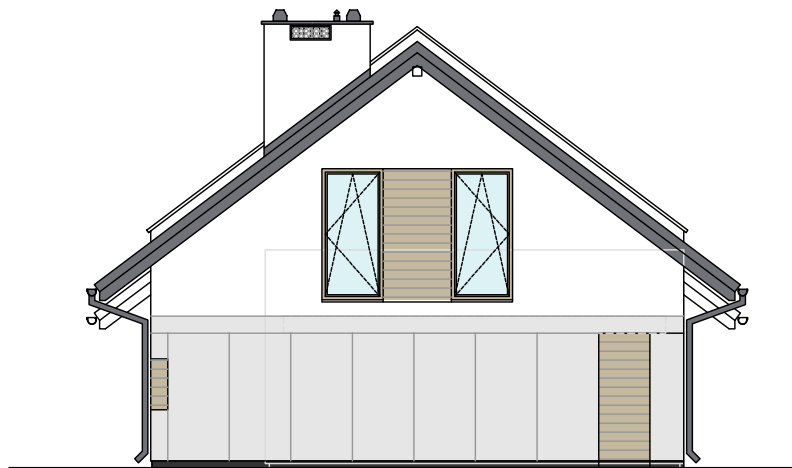
ELEWACJA ZACHODNIA
