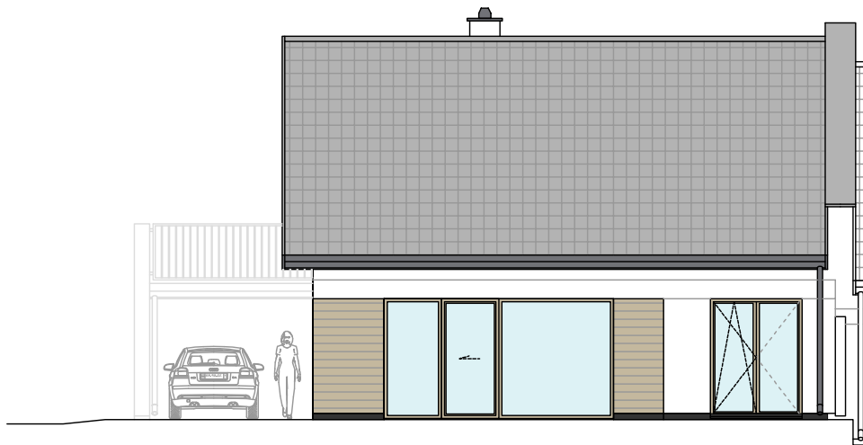
ELEWACJA POŁUDNIOWA
