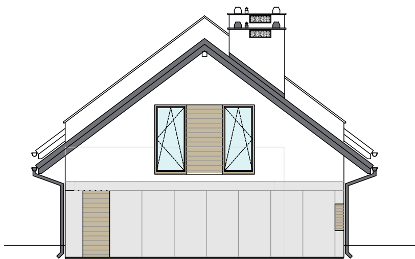
ELEWACJA WSCHODNIA
