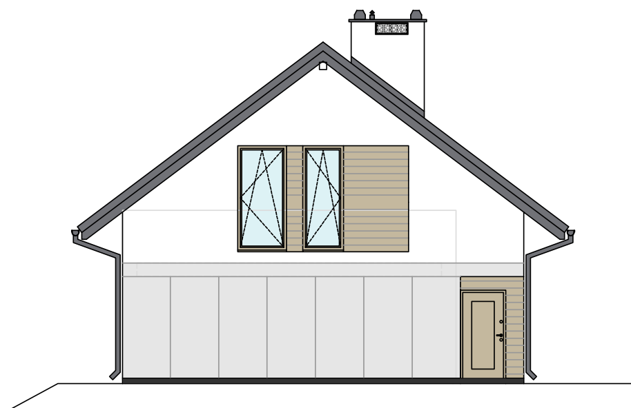
ELEWACJA WSCHODNIA
