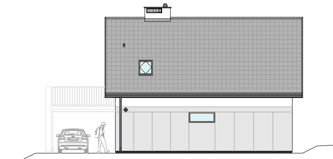
ELEWACJA PÓŁNOCNA
