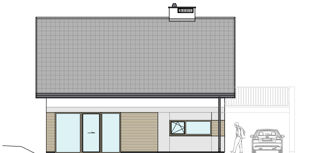
ELEWACJA POŁUDNIOWA
