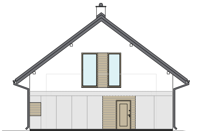
ELEWACJA WSCHODNIA
